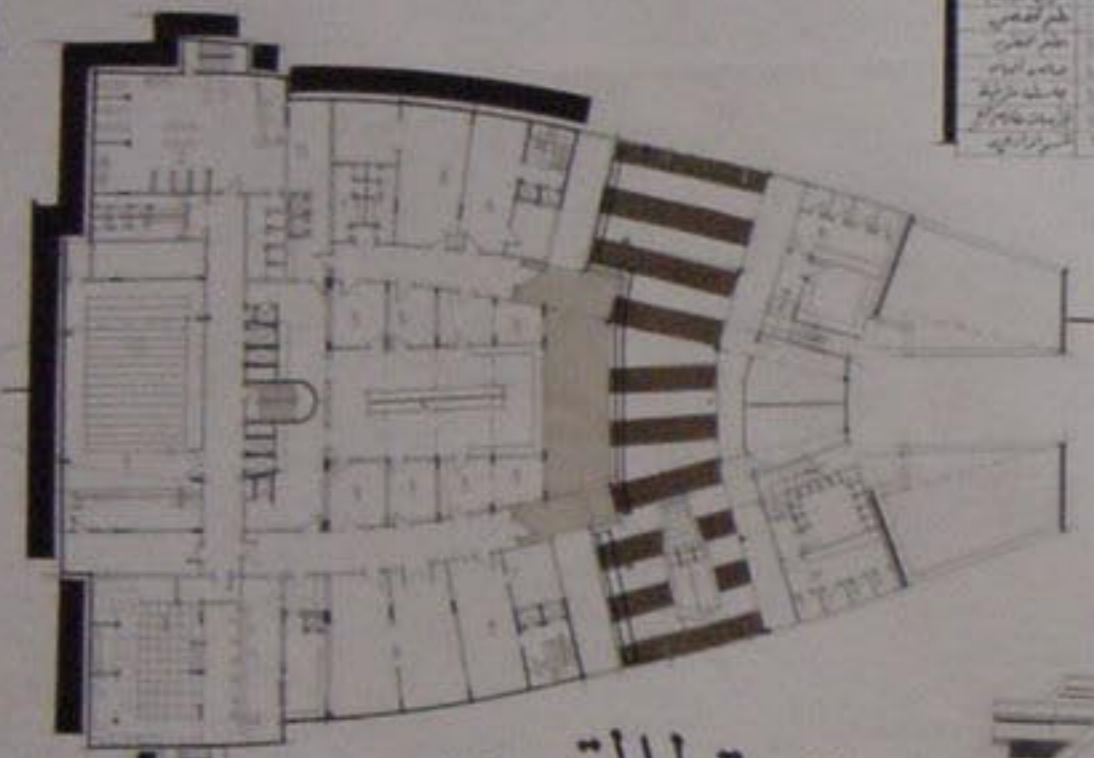
مسقط الطابق الاول ١/٢٠
