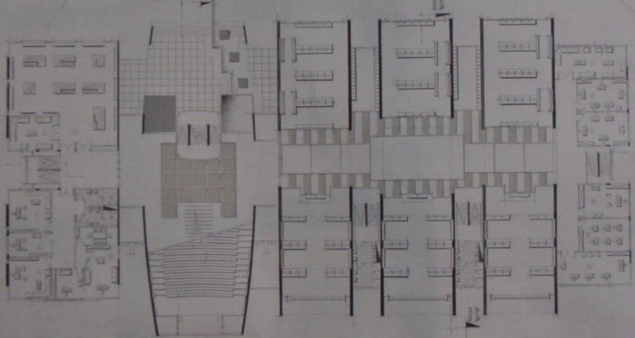
مسقط المنسوب ٣٧٥+ ١:١٠٠
