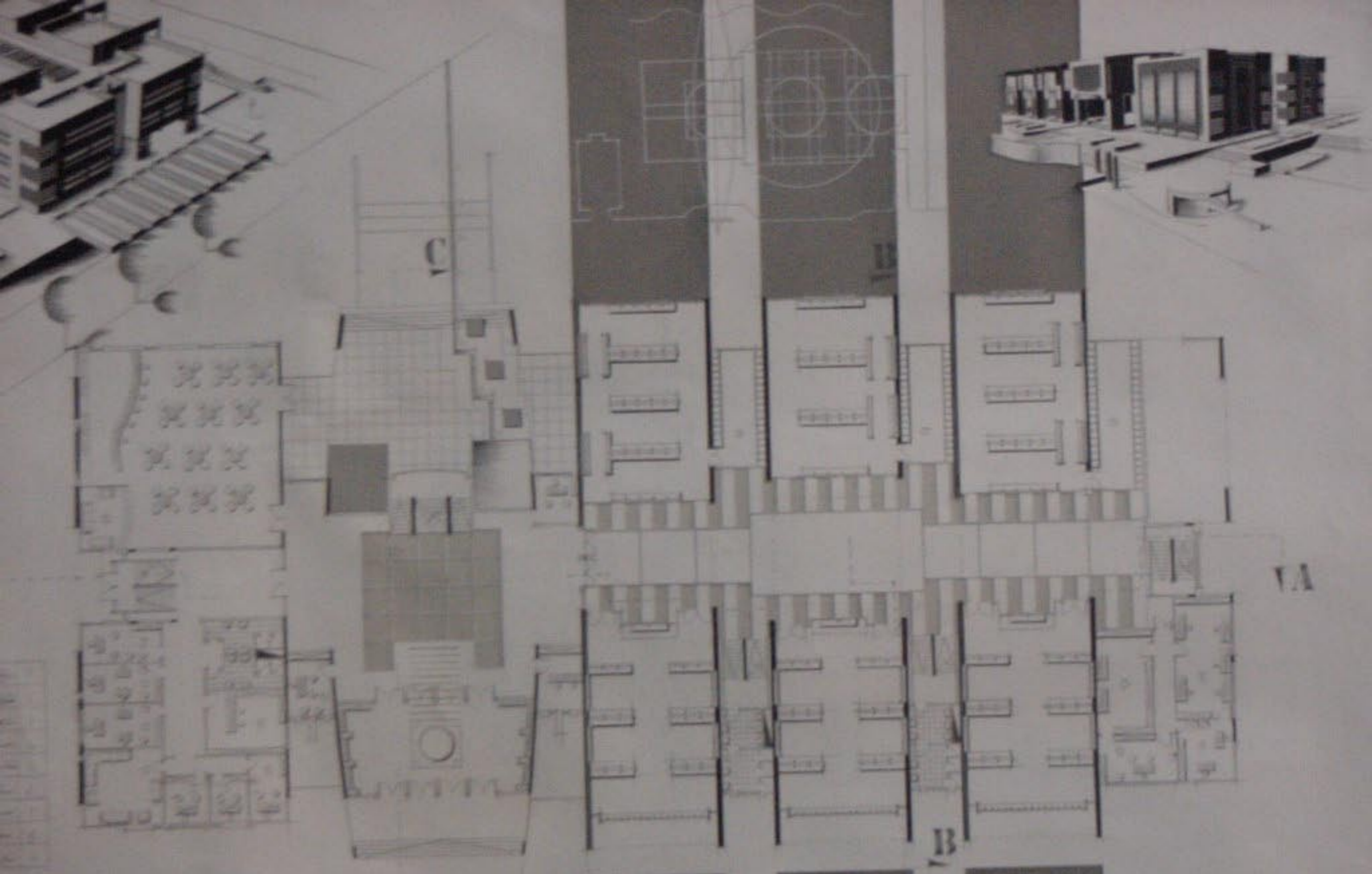
مسقط المنسوب ٧٥+ ١:١٠٠
