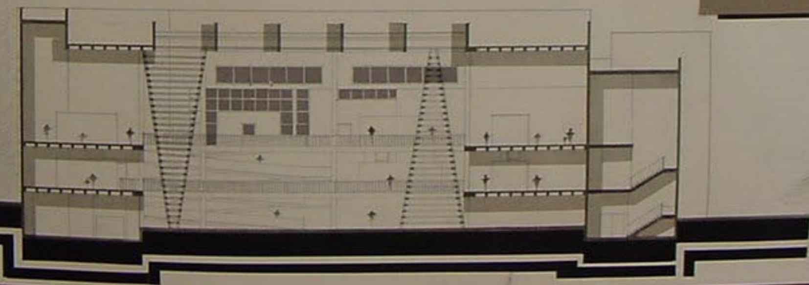
مقطع ١٠٠/١ م
