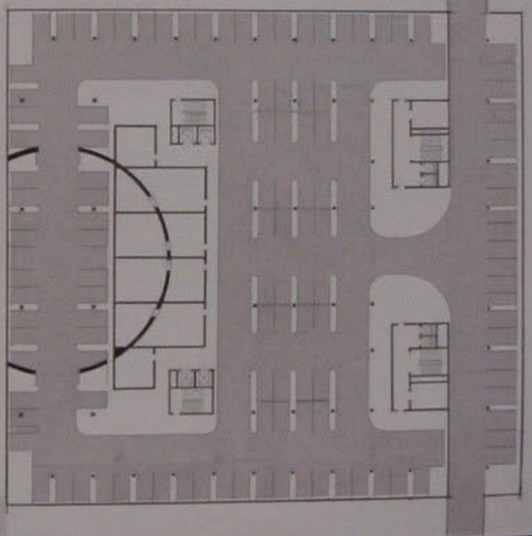
1/20 تفصيلة A-A
