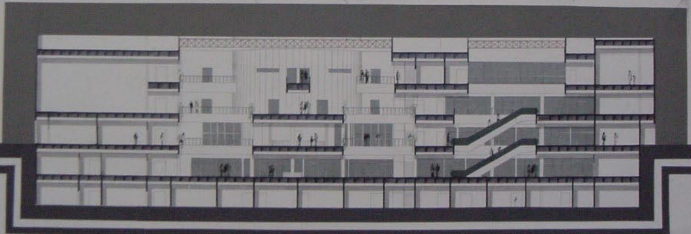
مقطع عمودي H-B ١٠٠١٦
