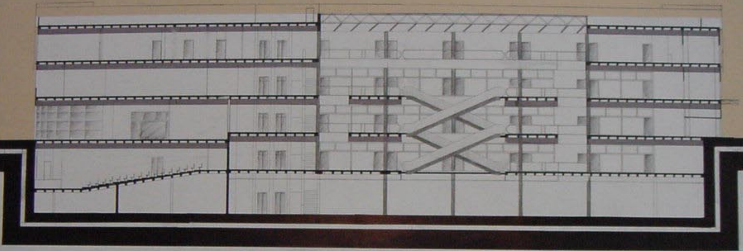
المقطع A - A 1/100
