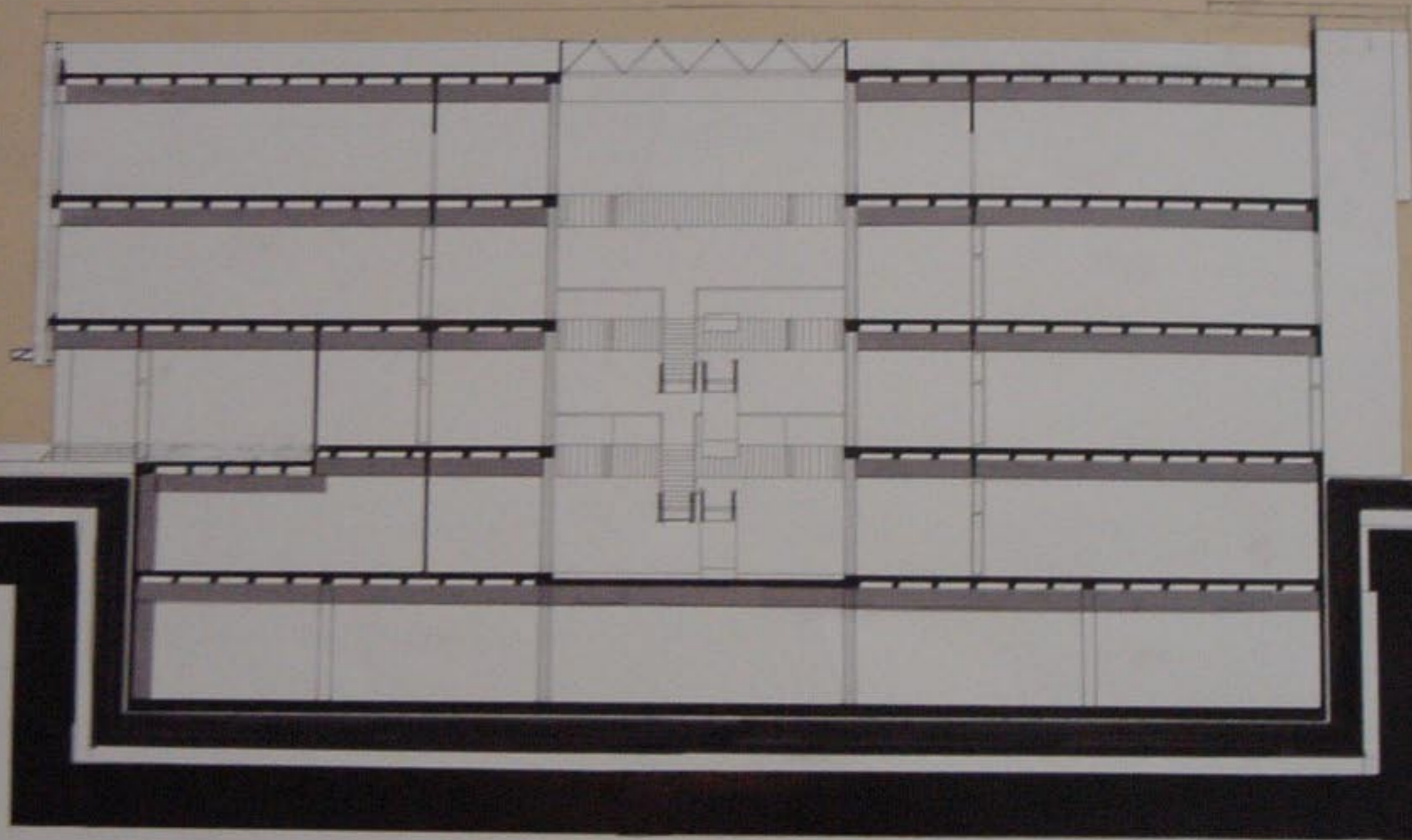
المقطع B-B 1/100
