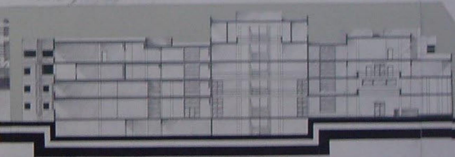
مقطع (2) مقايص 1/100
