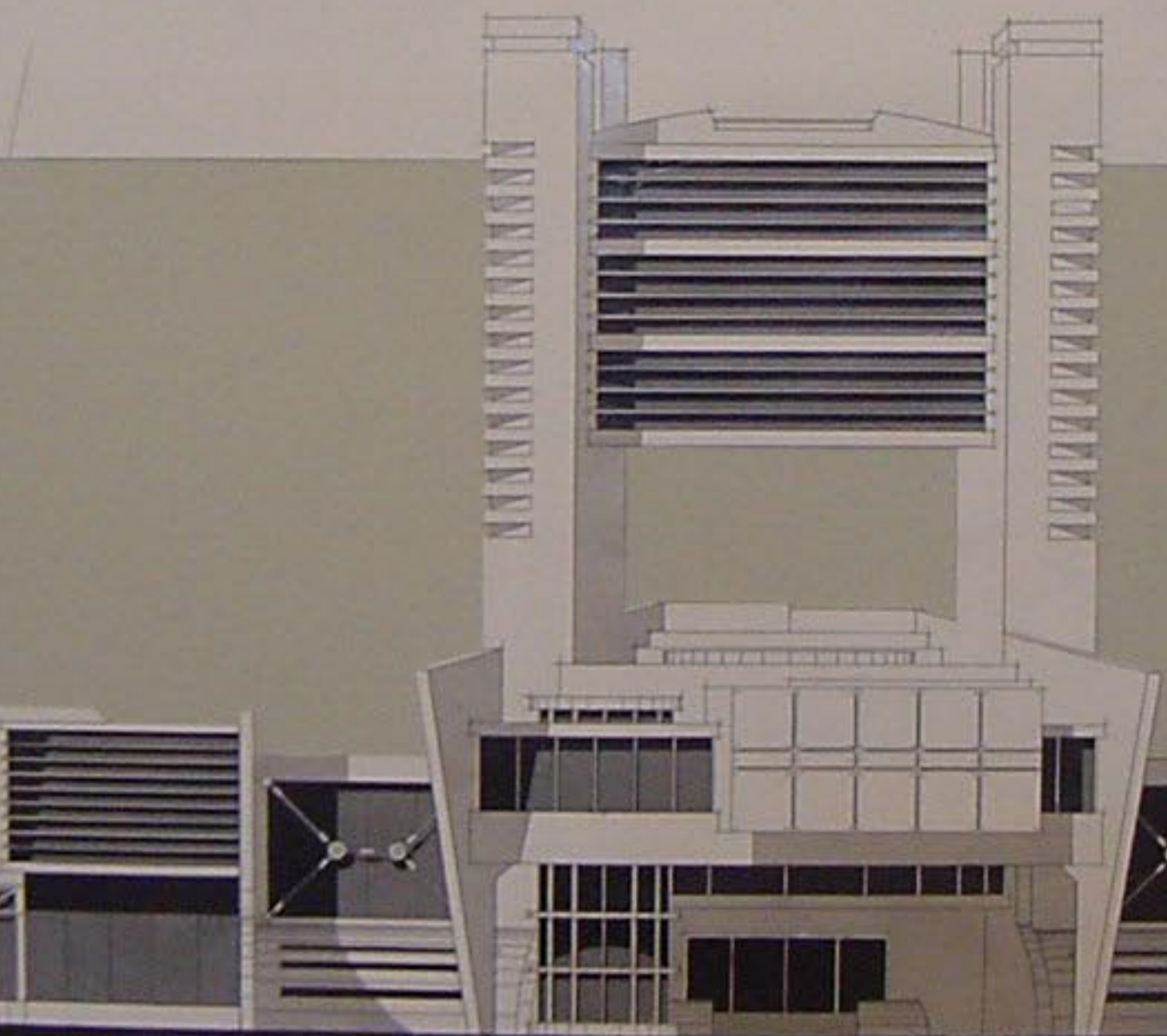
الواجهة الجنوبية مقايير 1/100
