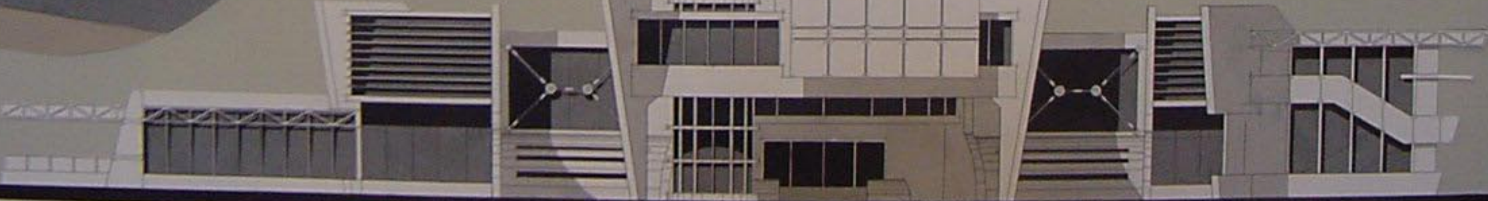
الواجهة الجنوبية مقايير 1/100
