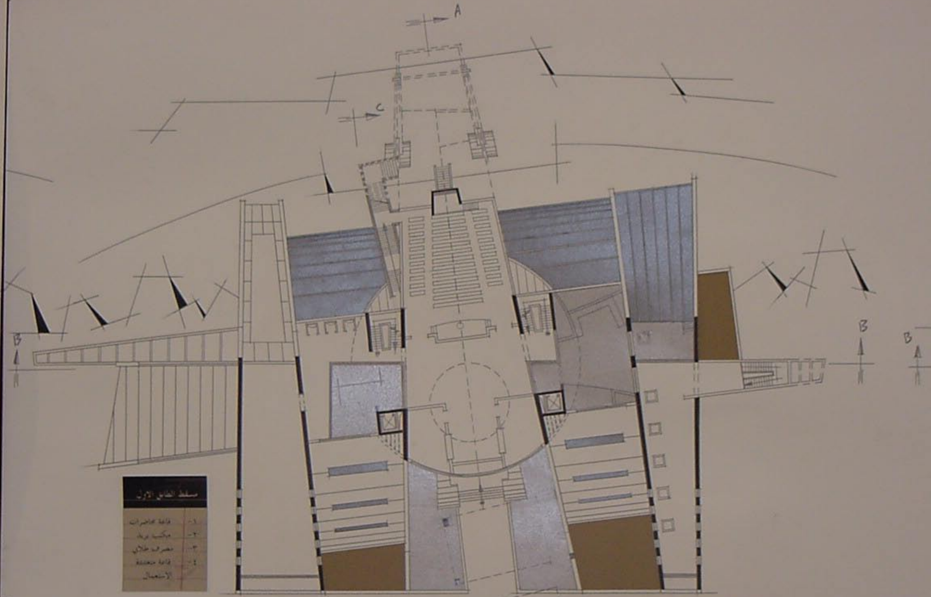
مسقط الطابق الاول مقياس 1/200 first floor
