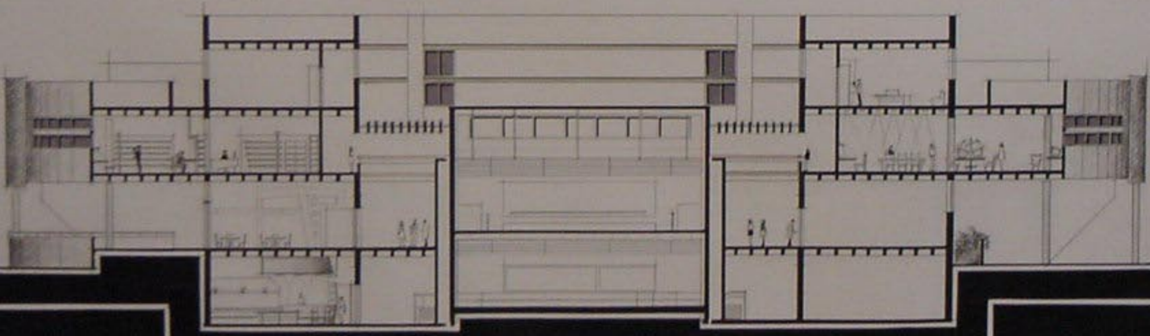
المقطع B-B ١/١٠٠
