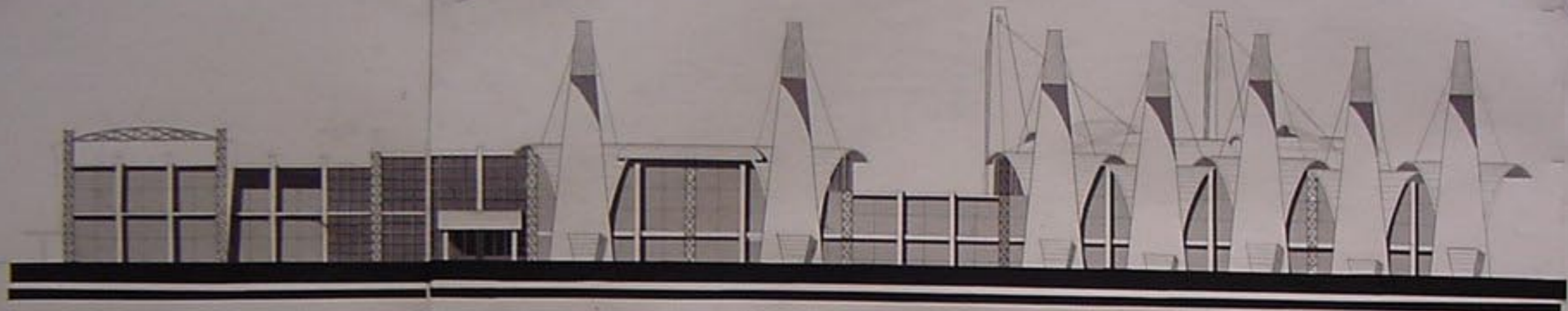
الواجهة الغربية ١٠٠/١
