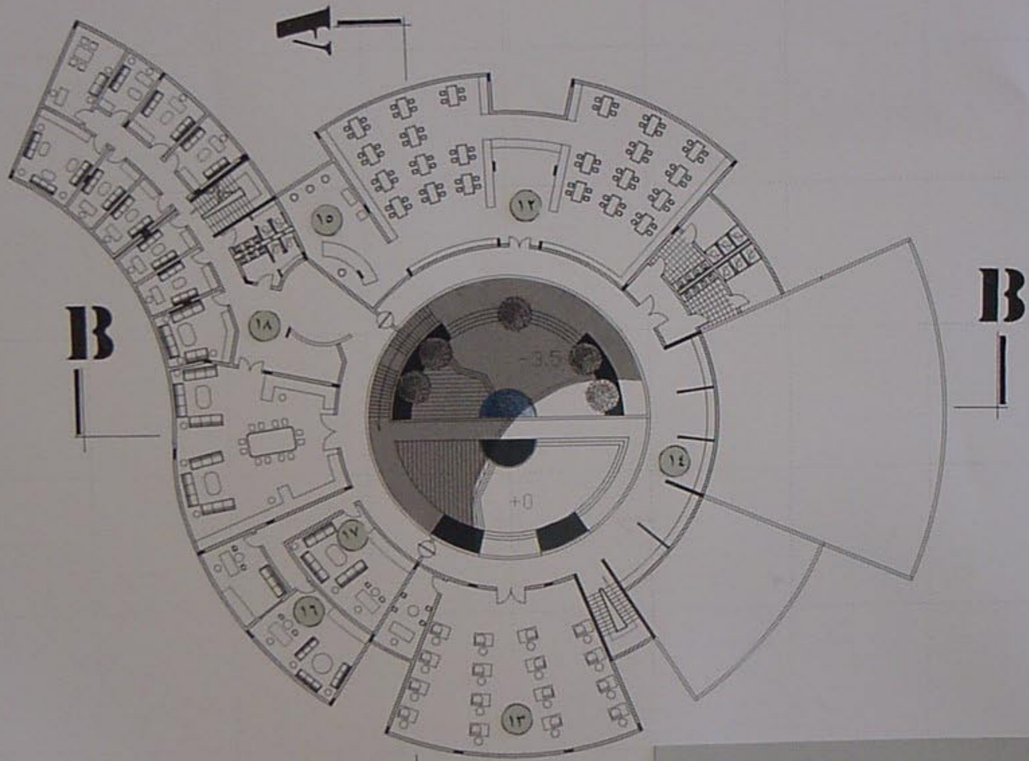
مسقط الطابق الثاني ١ : ٢٠٠
