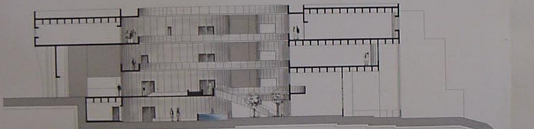
قطع A_A 1:100
